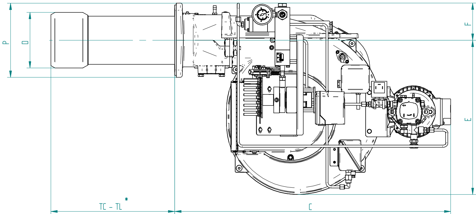
Fig. 3 Dimensions FGP 50/M EVO
