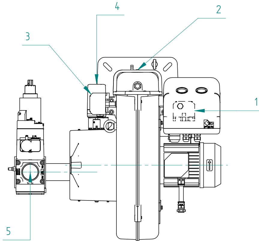
Fig. 13 РЕГУЛИРОВКА ГОРЕЛКИ
