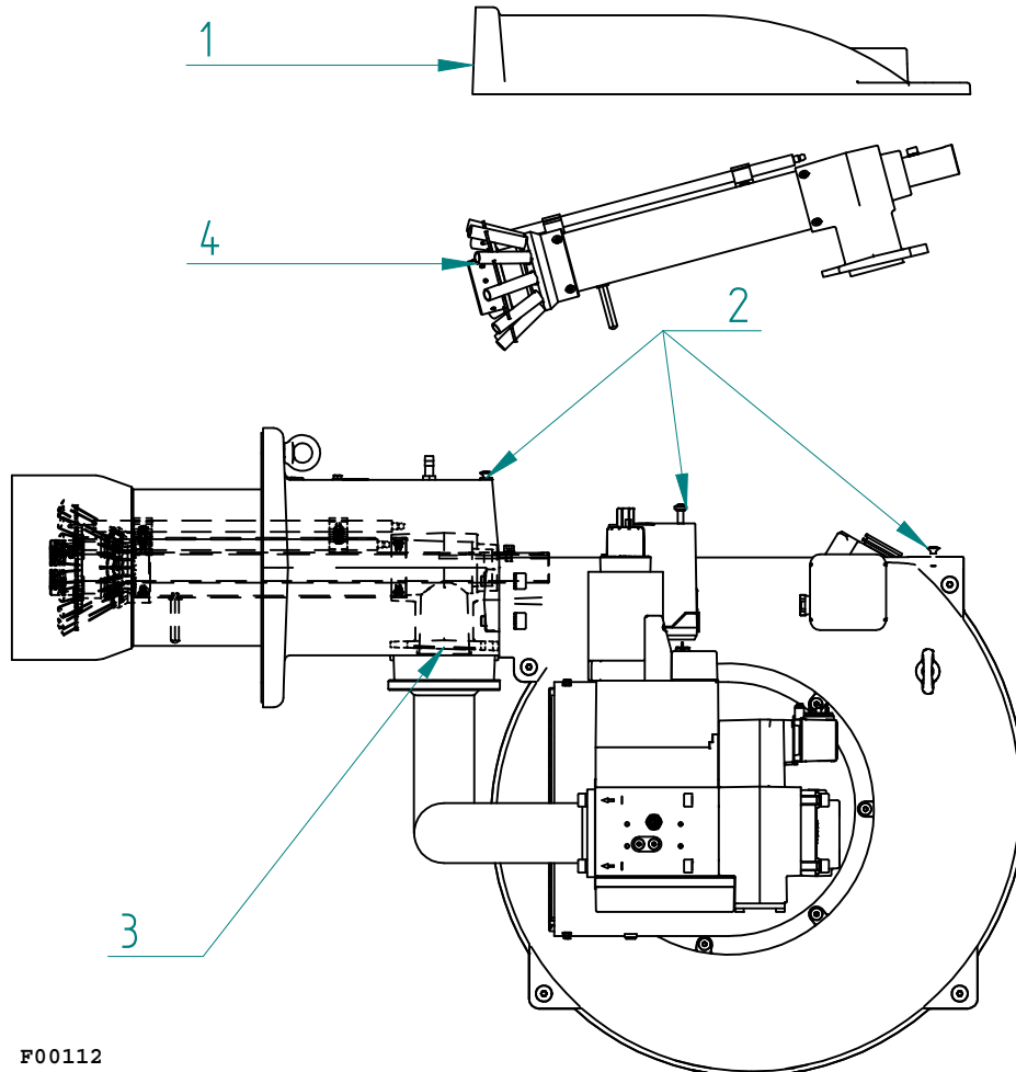
Fig. 17 ИЗВЛЕЧЕНИЕ СМЕСИТЕЛЬНОЙ КАМЕРЫ GAS P100/2 CE EVO
