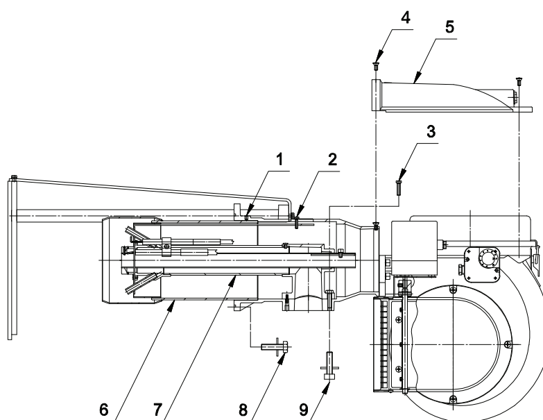
Fig. 19 ИЗВЛЕЧЕНИЕ СМЕСИТЕЛЬНОЙ КАМЕРЫ GAS XR80/2 CE - GAS P130/2 CE EVO - GAS P160/2 CE
