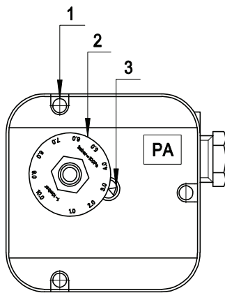
Fig. 14 1-Винт заглушка 2-Регулировочная гайка 3-Указатель регулировки
